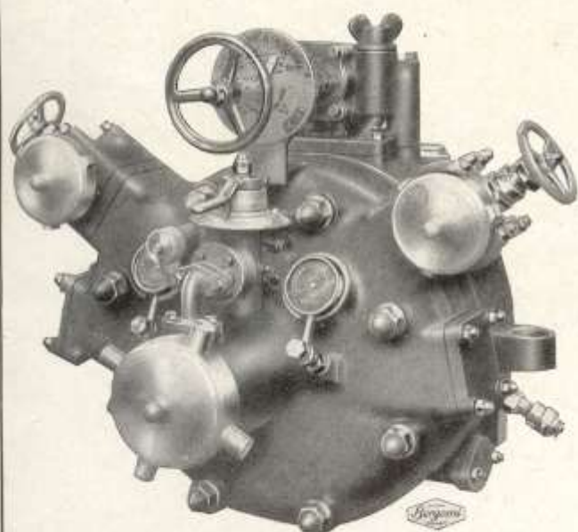
La pompa 1500/8
