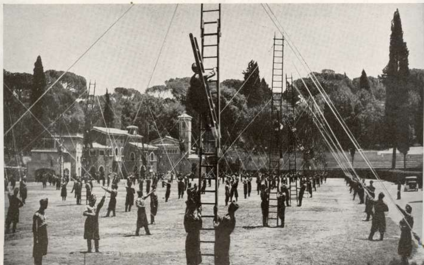
Scale italiane controventate: aggiunta della cima
